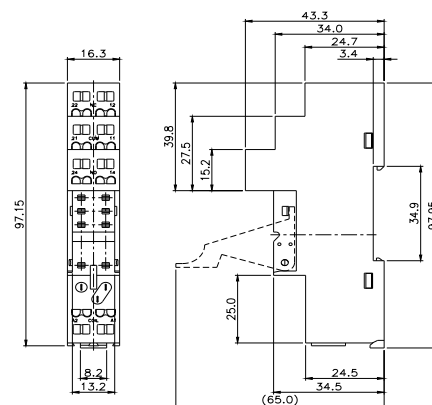
Module, Haltebügel
